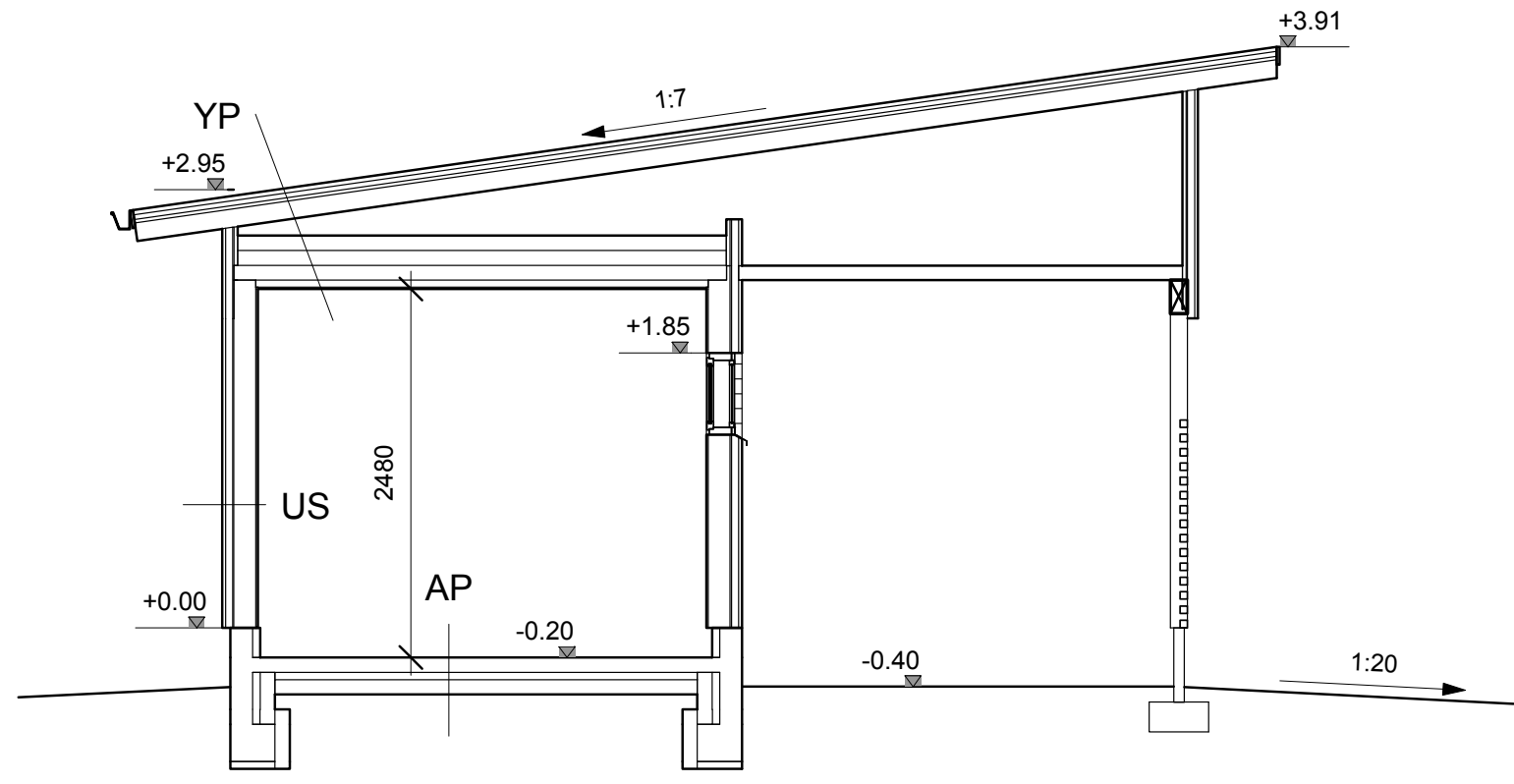
LEIKKAUS A-A
