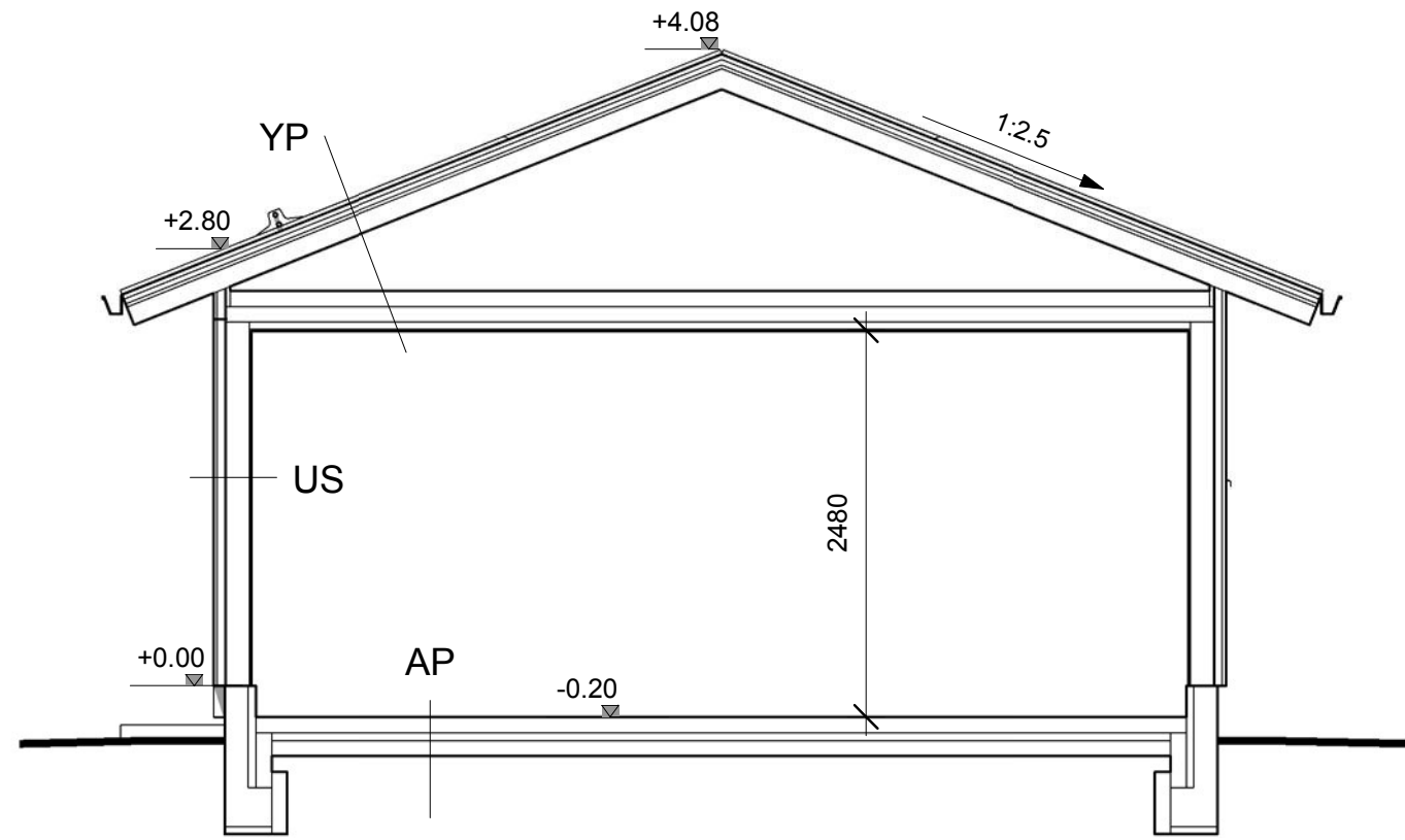
LEIKKAUS A-A
