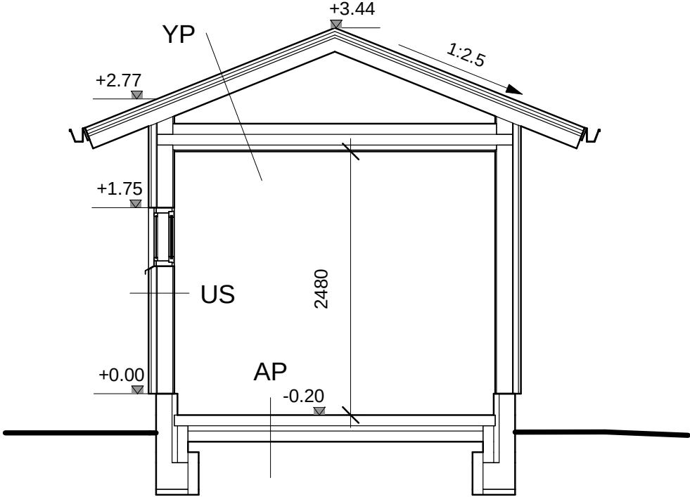
LEIKKAUS A-A
