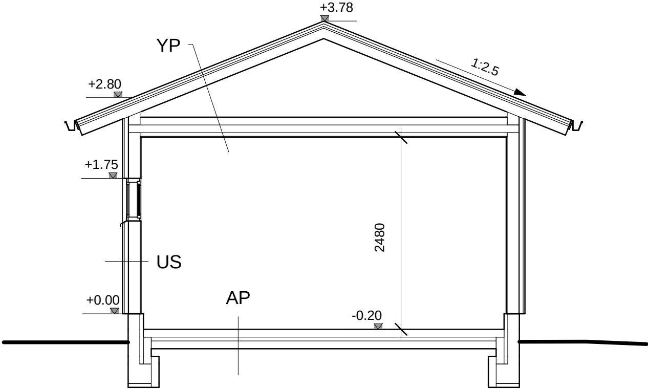
LEIKKAUS A-A
