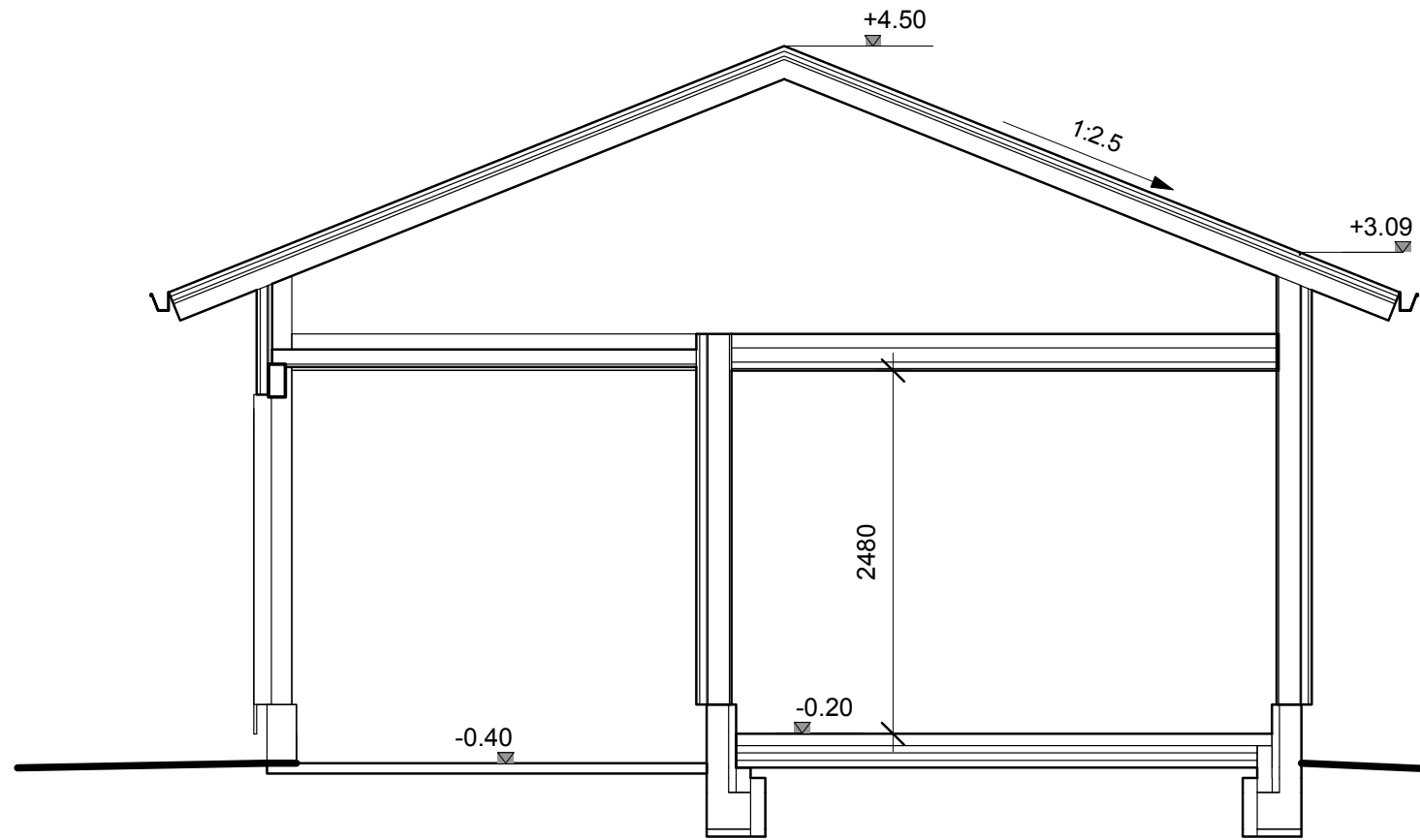
LEIKKAUS A-A
