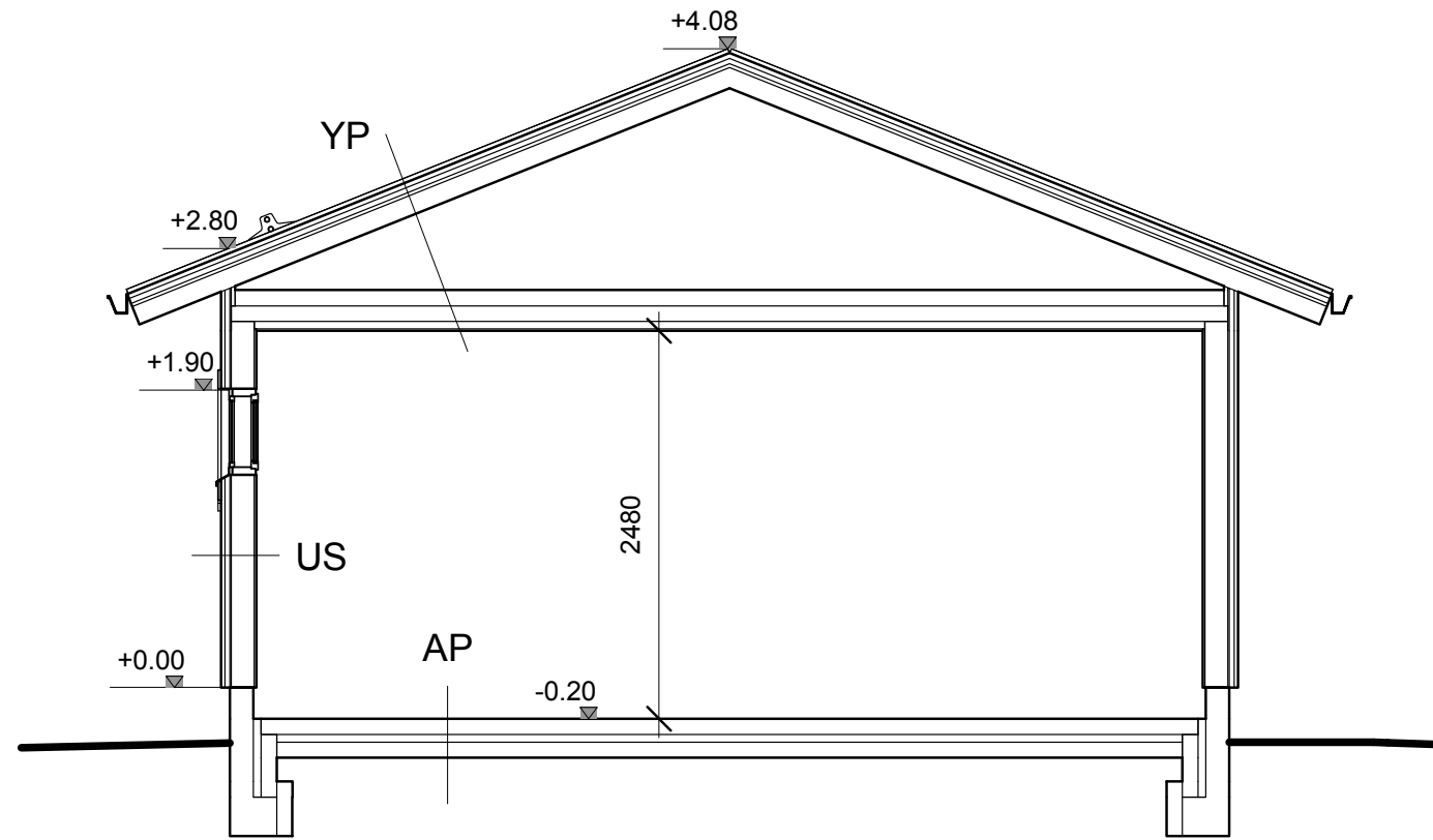
LEIKKAUS A-A
