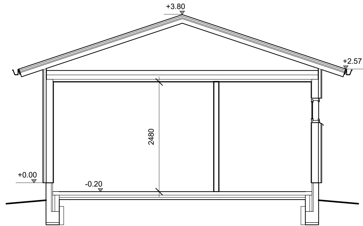
LEIKKAUS A-A
