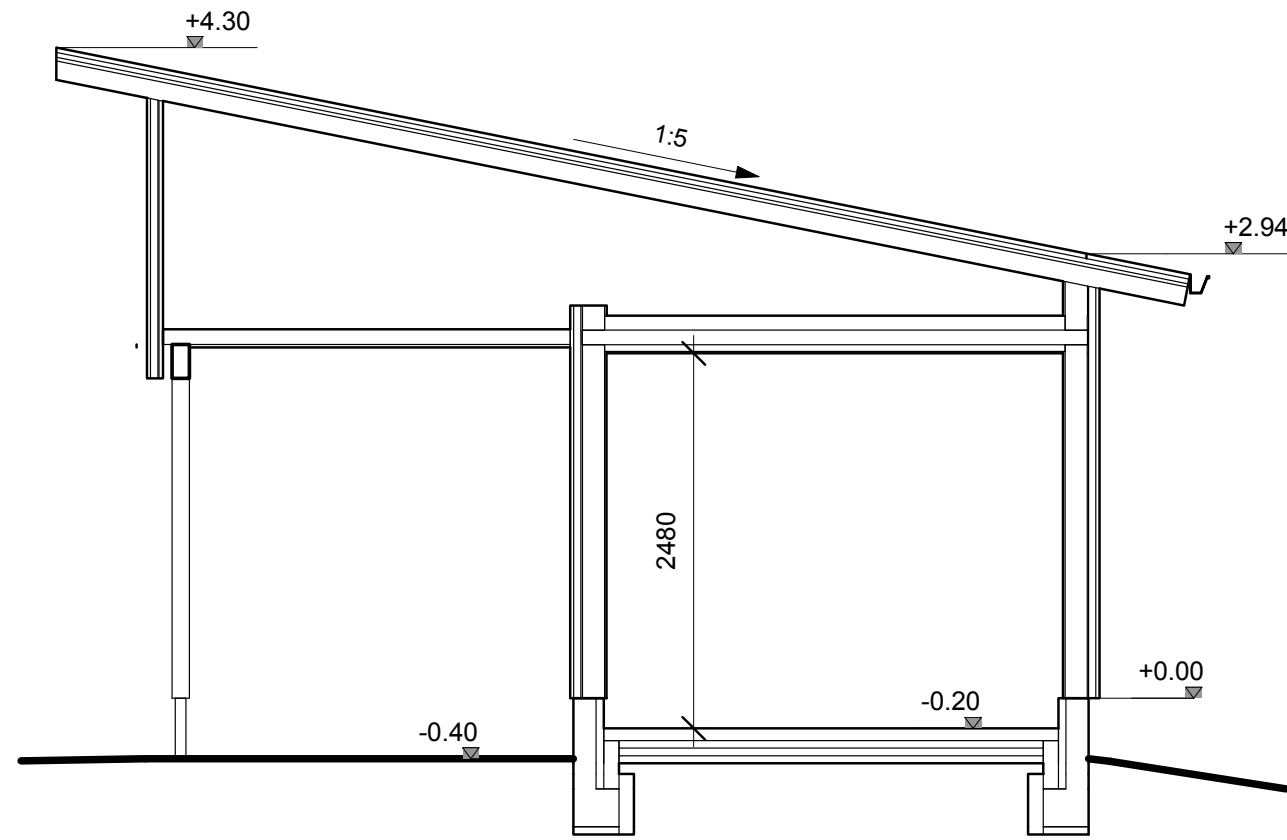
LEIKKAUS A-A
