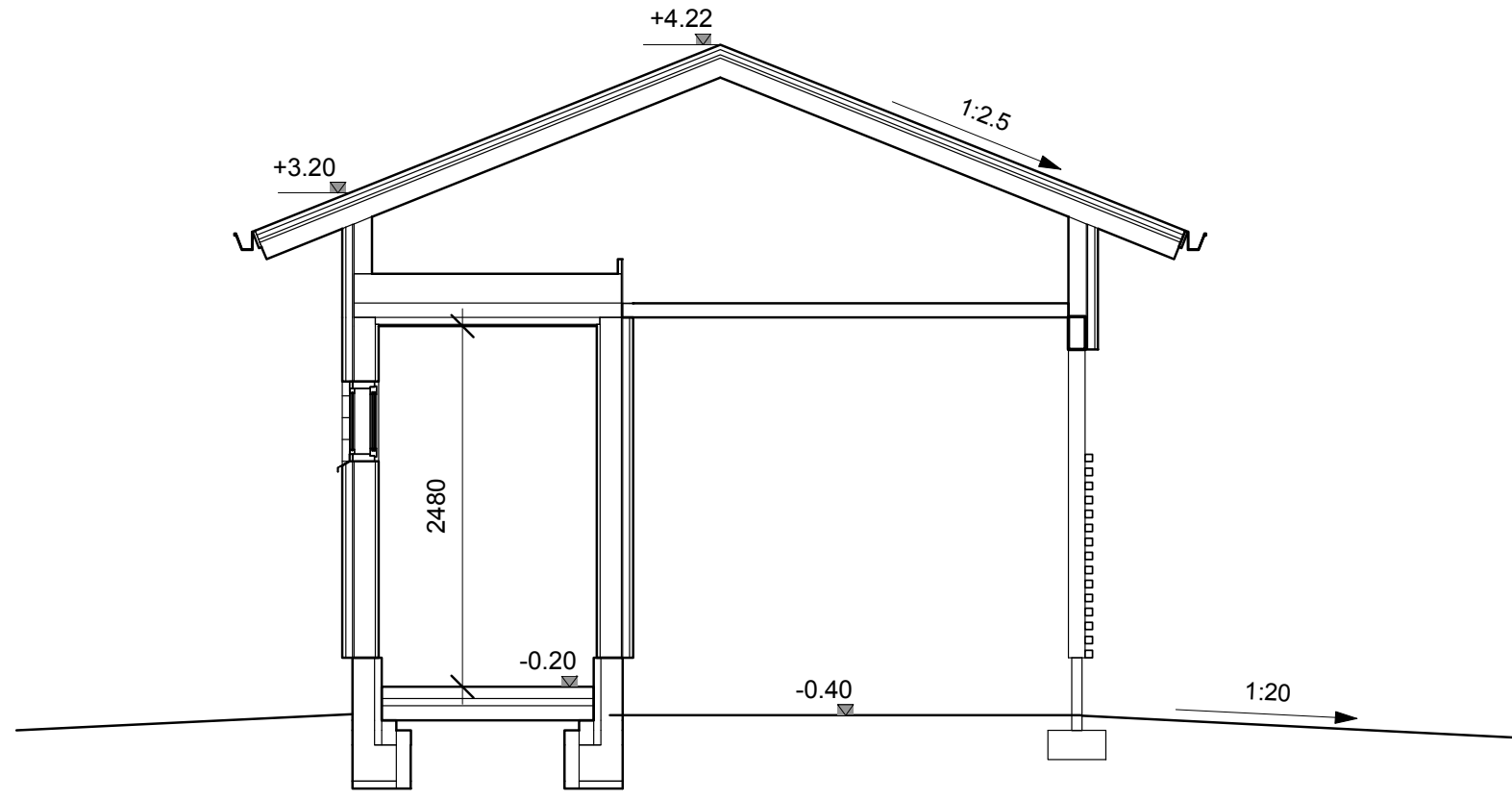
LEIKKAUS A-A
