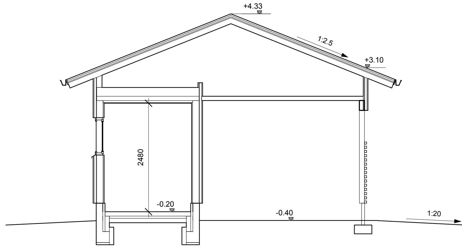
LEIKKAUS A-A
