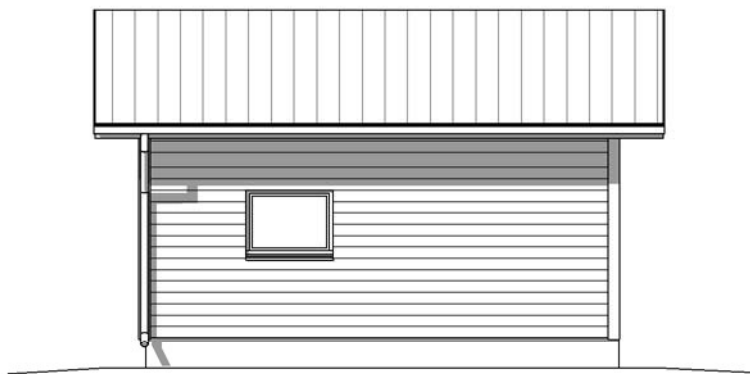
Sivu 2
