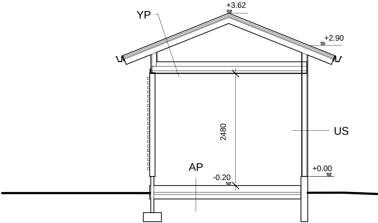
LEIKKAUS A-A
