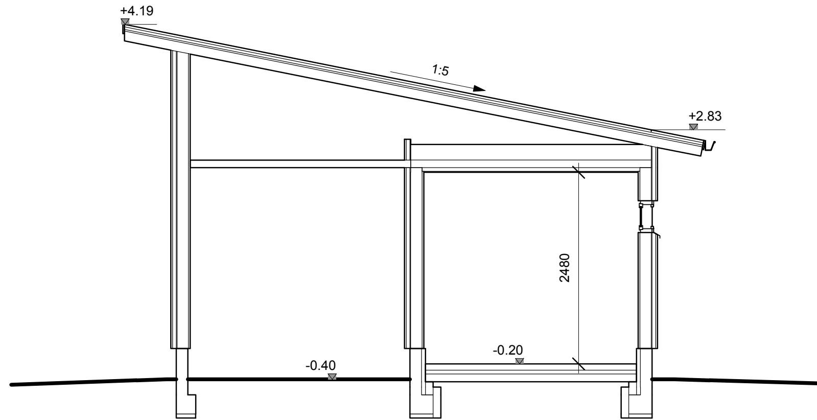
LEIKKAUS A-A
